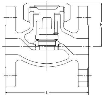
F-F dimension : JIS B 2002 JV 4-4 End flanges : JIS B 2239 20K
